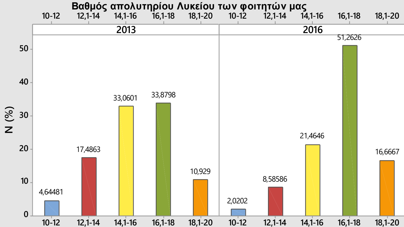
Chart of E38
